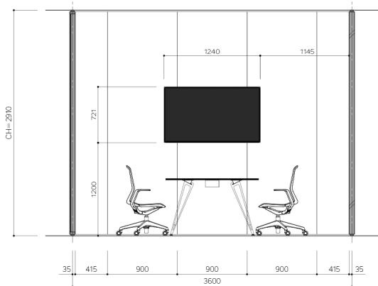
北側 展開図
