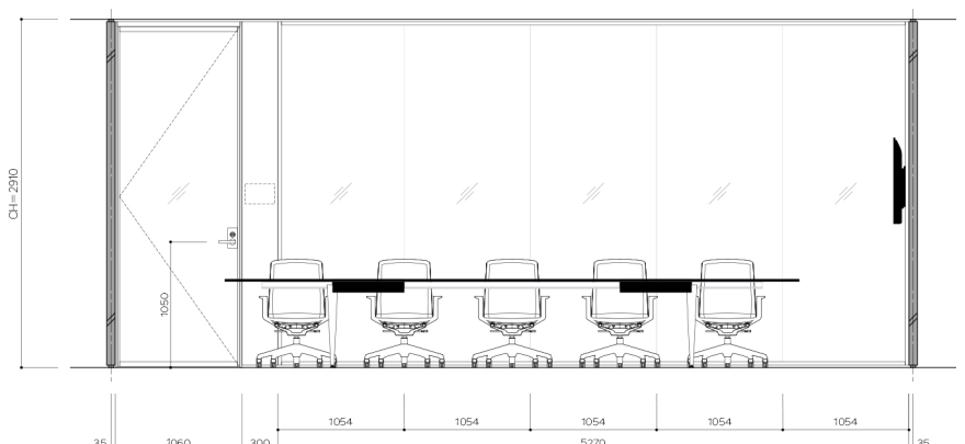
西側 展開図
