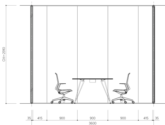
南側 展開図
